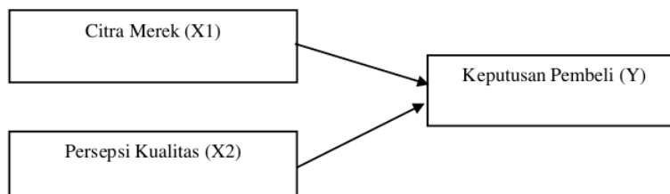
Gambar 1. Kerangka Analisis
