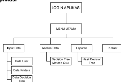
Gambar 5 Struktur Menu Aplikasi
