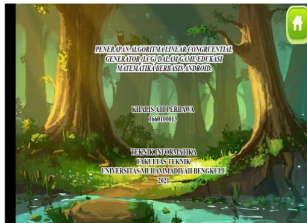
Gambar 7 Menu Tentang
