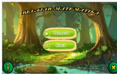
Gambar 2 Menu Utama
