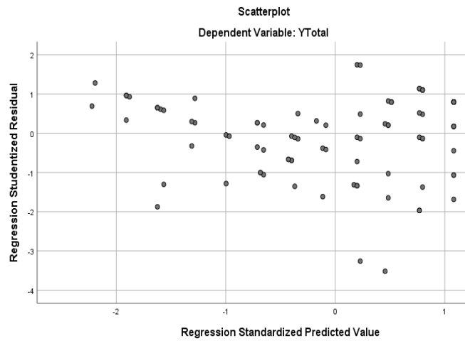
Gambar 1. Uji Heteroskedastisitas
